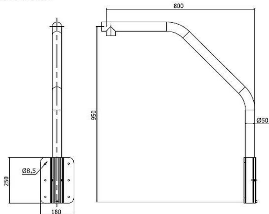
PM08 Dimensions
