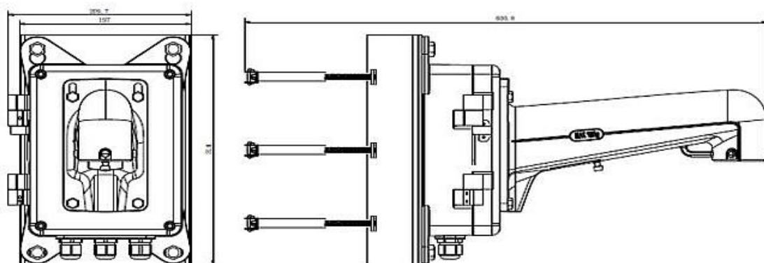
PM08 Dimensions
